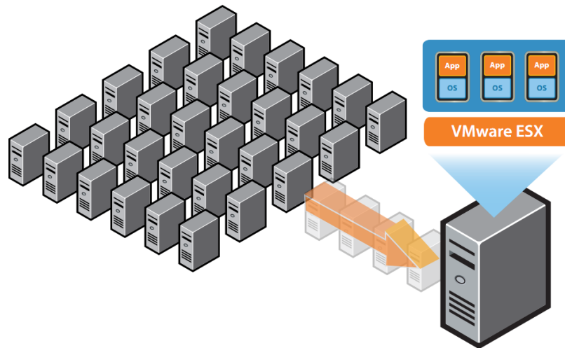
Abbildung 3: Konsolidierung durch Virtualisierung. Mehrere leistungsschwache und selten ausgelastete Server werden auf einem leistungsstarken Server konsolidiert. Alle konsolidierten Server laufen dann in einer virtuellen Maschine auf dem leistungsstarken Server und werden vom Hypervisor (hier: VMware ESX ) verwaltet. Quelle: (VM08)
