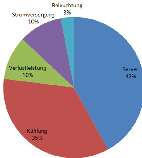
Abbildung 1: Eine ungefähre Zusammensetzung der Faktoren, die beim Energieverbrauch eines Rechenzentrums von Bedeutung sind. Werte entnommen aus (BGa09; SPa09)
